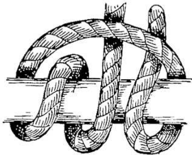
FIG. 49.—Magnus hitch.
